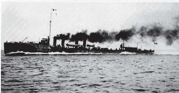
La DAGUE, d'une série de 13 contre-torpilleurs, déplaçait 715 tonnes et était armée de 2 canons de 100, de 4 pièces de 65 et de 4 tubes lance-torpilles. (Service historique de la marine - Collection Doussier).
